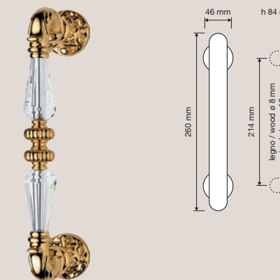
1542 MN 214 Maniglione. Attenzione: l'interasse può variare leggermente, chiedere sempre le misure prima di forare la porta. / Pull handle. Attention: the distance can have little changes, please always ask before making the holes in the door.
